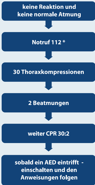
Abb 1.3.: Der BLS-AED-Algorithmus
